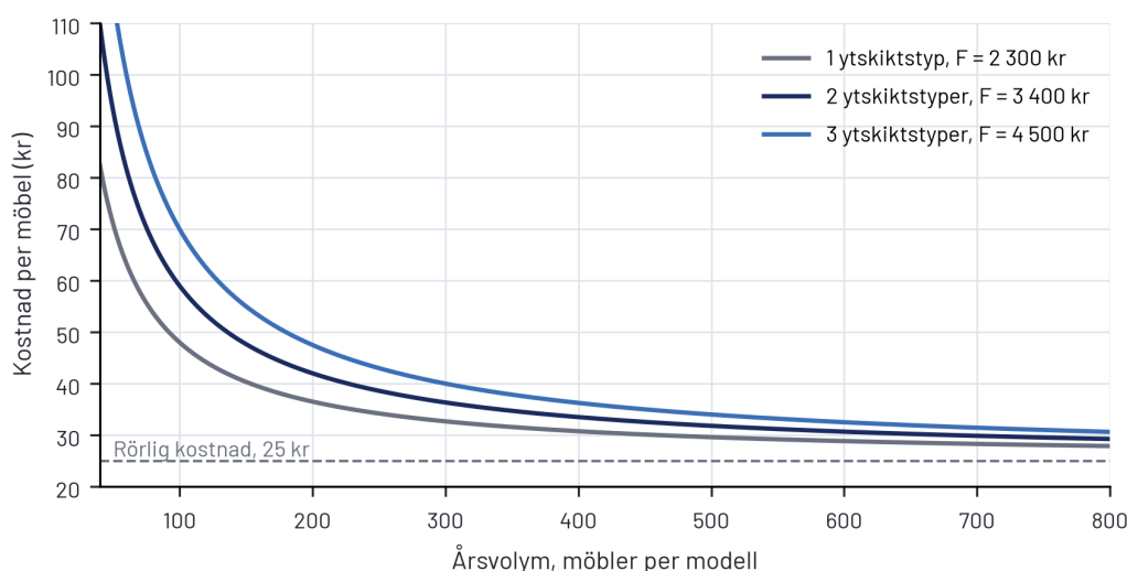
Figur 2. Kostnad per möbel som funktion av årsvolym för modeller med ett, två och tre ytskiktstyper
